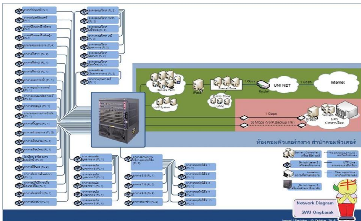
แผนภาพ 3 : การเชื่อมต่อเครือข่ายบัวศรี มหาวิทยาลัยศรีนครินทรวิโรฒ องครักษ์
